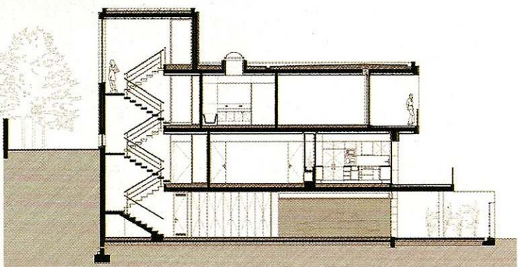
corte
