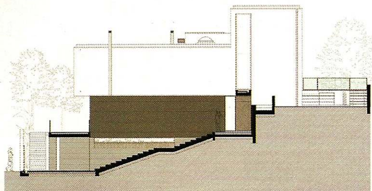
alçado Sul
